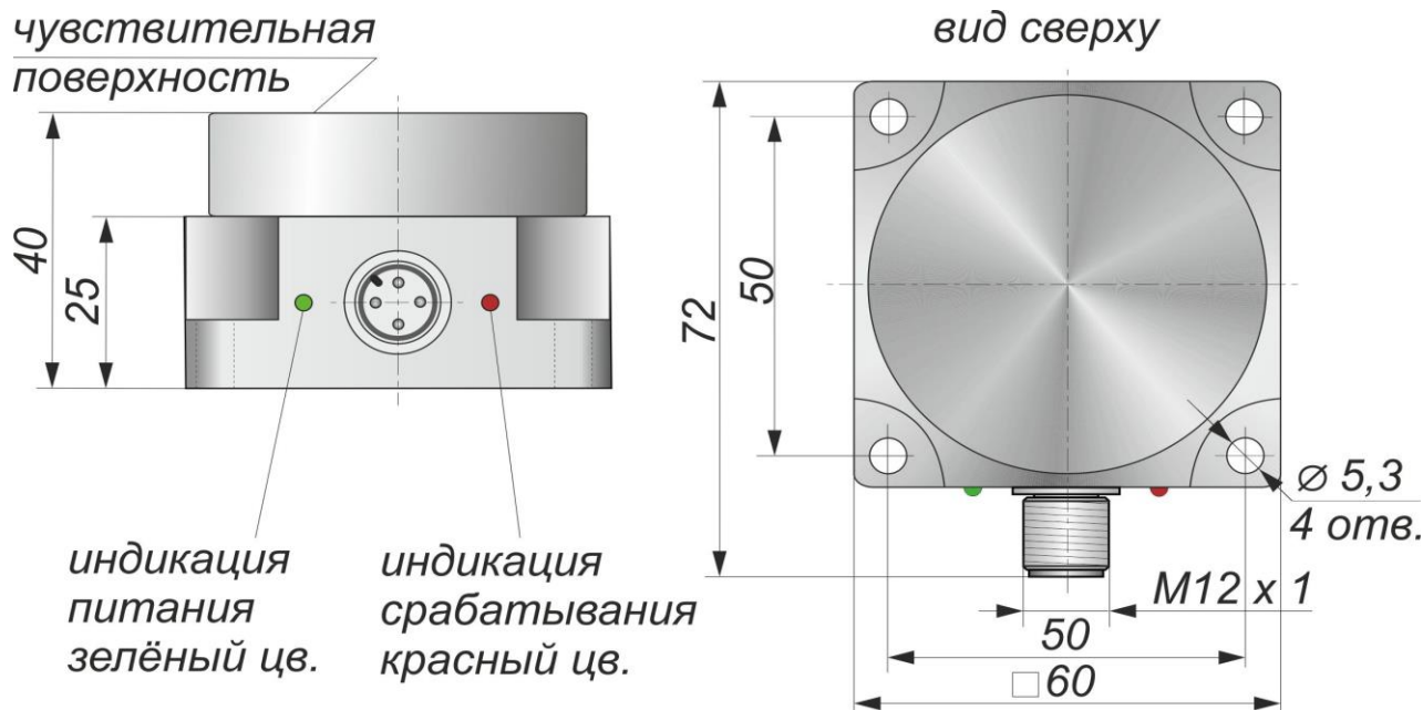
Габаритный чертеж
